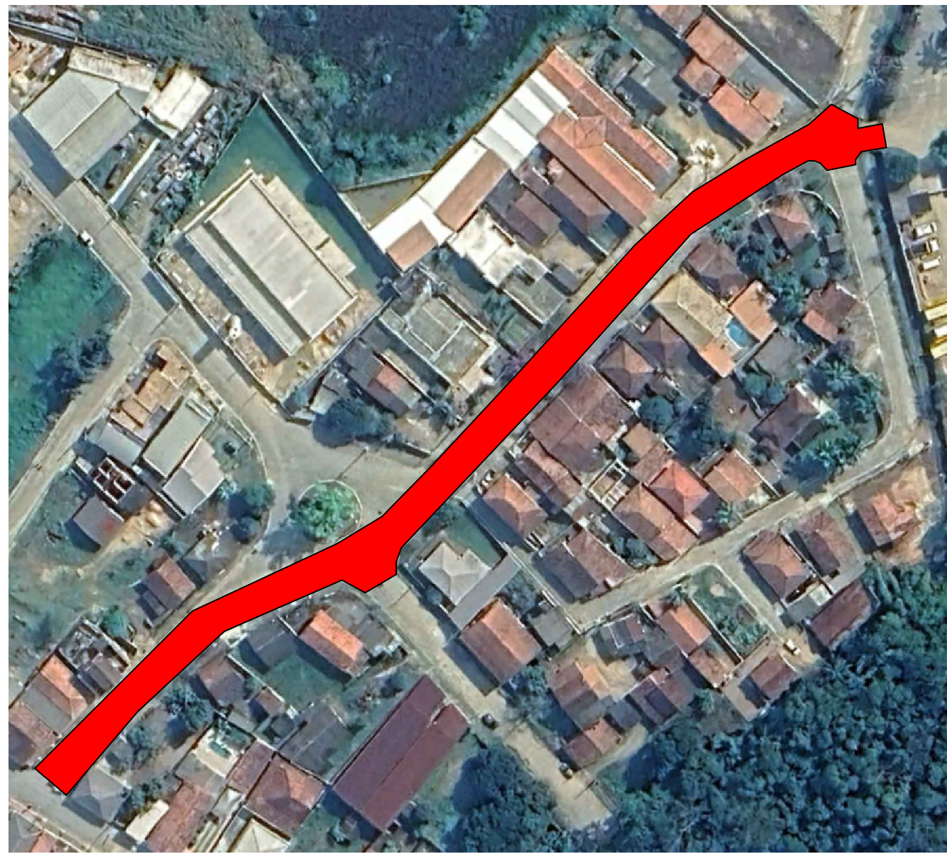
Implatação Geral Rua Herculino da Silva Rosa Esc: 1:300
