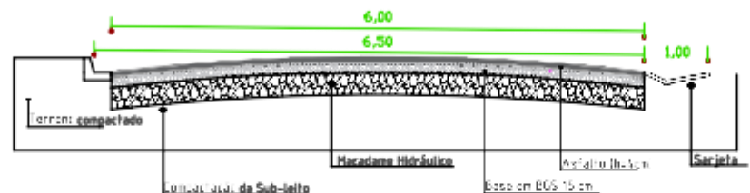
Corte Genérico 2 Sem Escala
