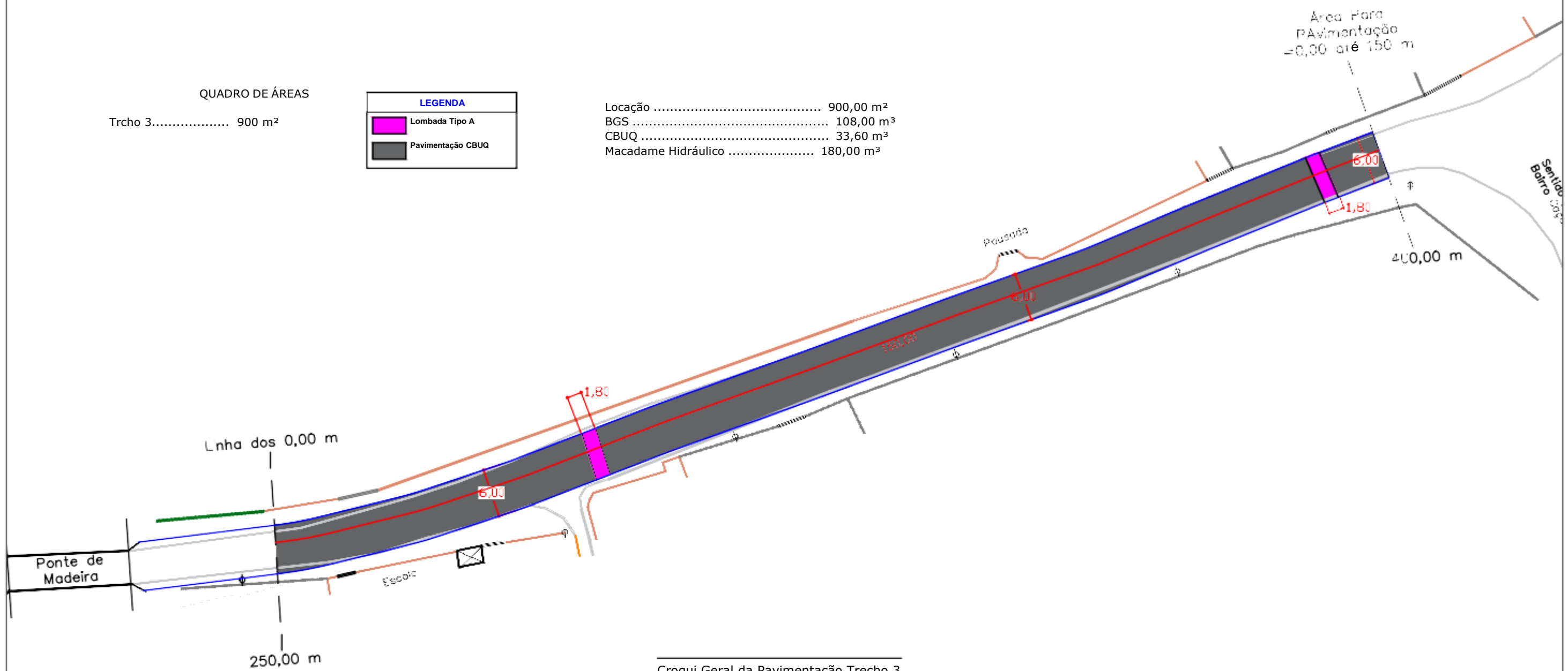
Croqui Geral da Pavimentação Trcho 3 Esc. 1:200
