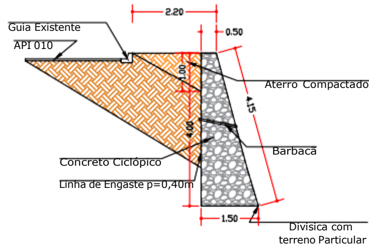
Corte-AA Escala: 1:100
