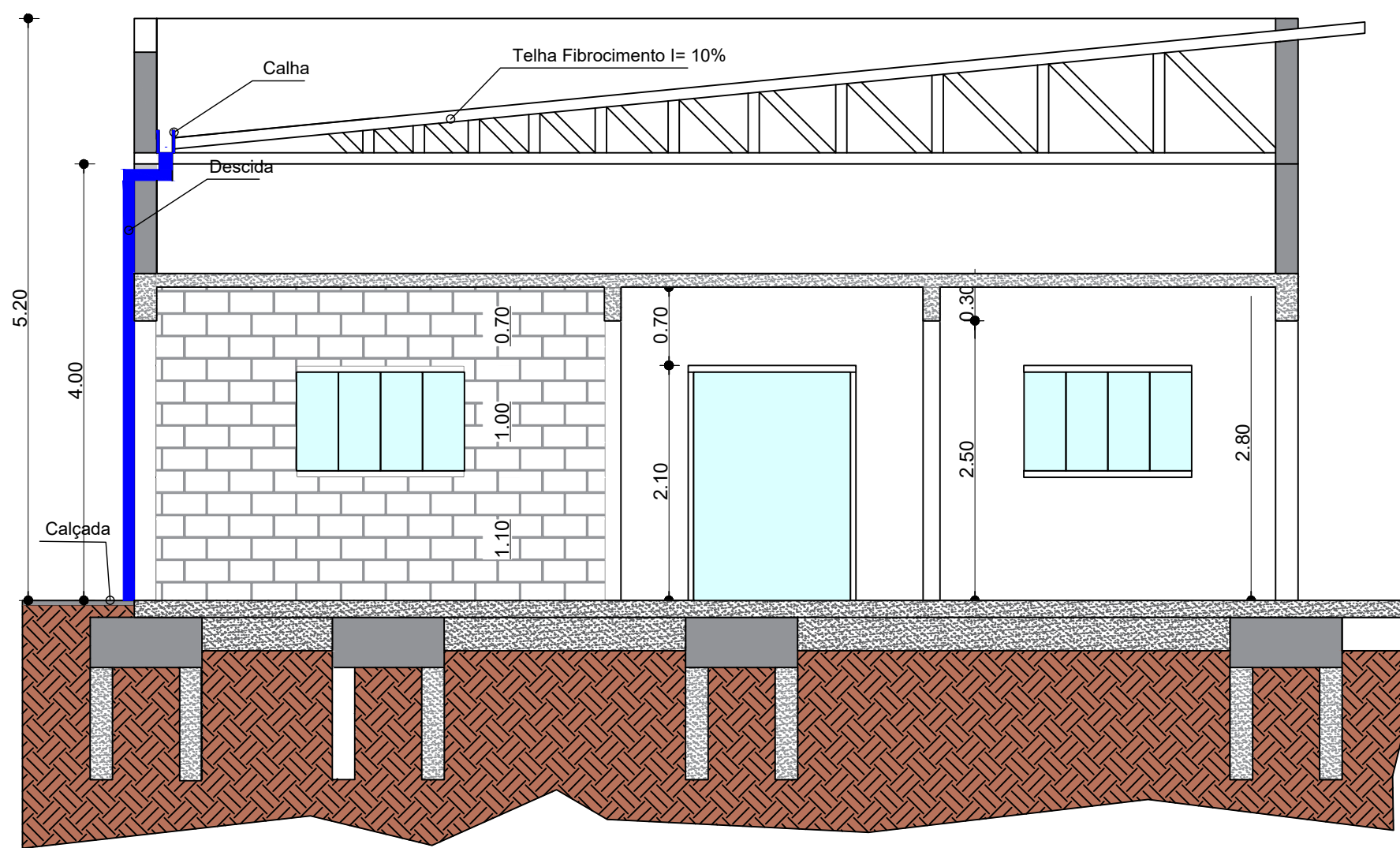
Corte AA ESCALA DETERMINADA
