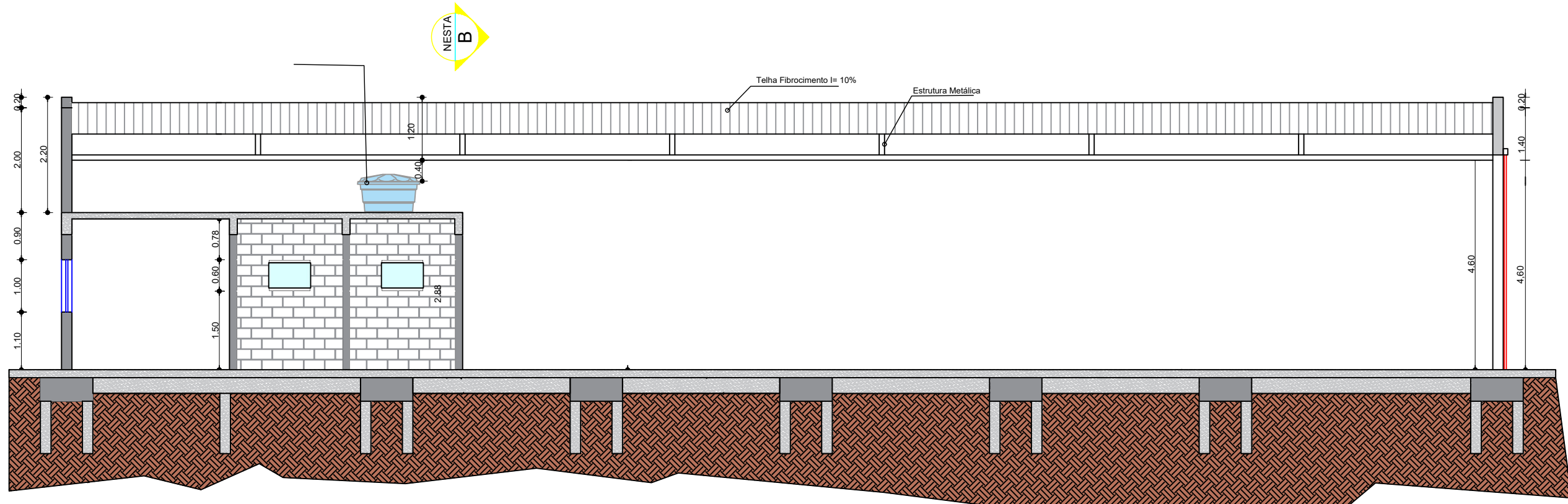
Corte BB ESCALA DETERMINADA
